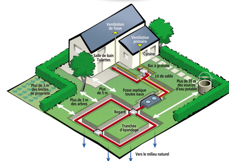
Installation d'un système d'assainissement non-collectif
